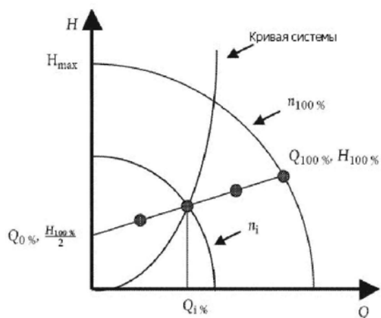
Рис. 2. Кривая системы интегрированного циркуляционного насоса.
